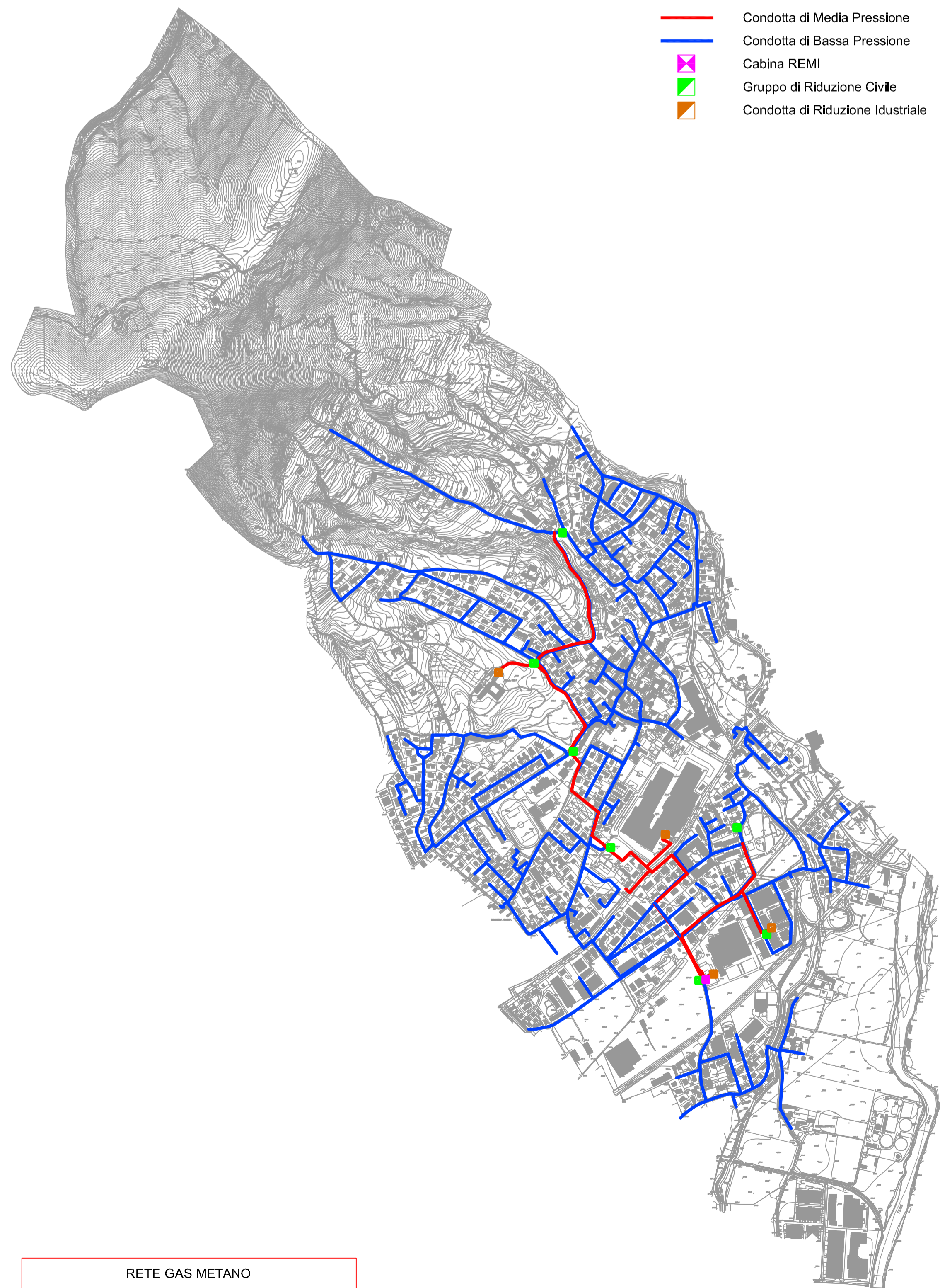
RETE GAS METANO
